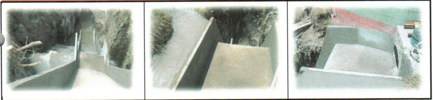
30. CONSTRUCCION MURO DE CONTENCION, PARAJE CHONIMACORRAL, ALDEA SAN ANTONIO SIJA, SAN FRANCISCO EL ALTO, TOTONICAPAN
